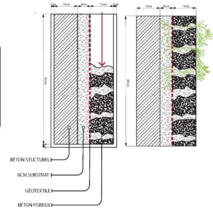
ÉTAPE 2 MOULAGE VERTICAL
