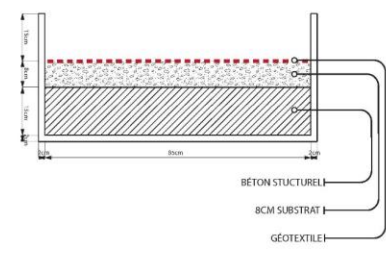
ÉTAPE 1 MOULAGE HORIZONTAL
