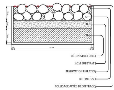
ÉTAPE 1 MOULAGE HORIZONTAL
