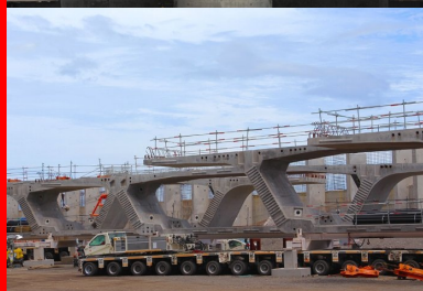
Stockage de voussoirs sur le site de pose. Le tablier est découpé en 1 206 voussoirs préfabriqués sur une aire dédiée de 9 ha à quelques kilomètres du chantier.
