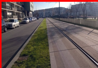
La plate-forme du tramway T6 est constituée d'une dalle courte en béton non armé et goujonné.
