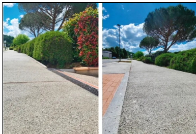
Ph 13. Désimperméabilisation et aménagement d'espaces publics piédonniers, chemin de la Gardie au Séquestre (81). Ciment utilisé : CEM III/B. © LAFARGE
