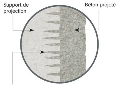
Incrustation de la couche d'accueil du béton projeté dans les pores du support
