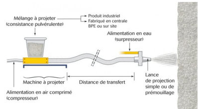
● Schéma de projection par voie mouillée (source : Infociments.fr)
