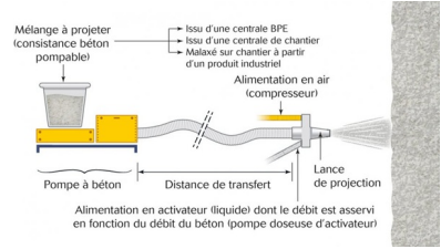
● Schéma accrochage mécanique du béton projeté par voie sèche sur le support (source infociments.fr)
