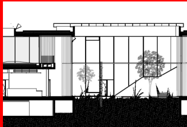
Coupe sur le Patio
