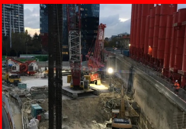
La cage d'armature est placée au-dessus de la tranchée, avant d'être descendue avec précaution jusqu'au fond.
