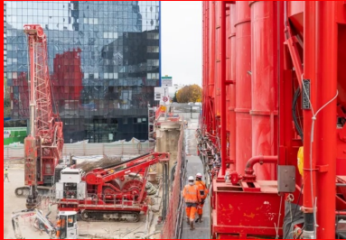
La boue bentonitique est traitée pour en éliminer les particules solides et les impuretés, puis elle est stockée jusqu'à ce qu'elle soit prête à être réutilisée. Ce processus en circuit fermé permet d'économiser de l'eau, de la bentonite et de réduire les coûts de traitement des déchets.
