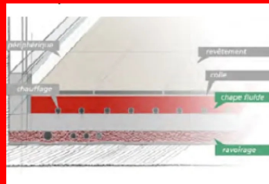
Exemple de ravaillage pour une chape fluide
