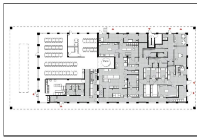
Plan rez-de-chaussée
