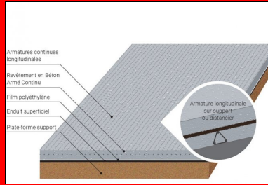
Vue en perspective de la structure réalisée sur le chantier d'Escaliers : largeur 4 m et structure sans fondation.
