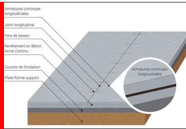
Vue en perspective d'une structure en BAC : cas général pour une largeur supérieure à 5 m et une structure avec fondation
